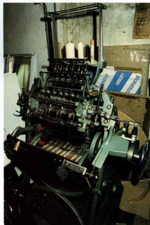
↑ Máquina de coser de hilo vegetal.
